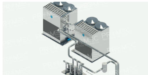
Modelado BIM (HVAC)
